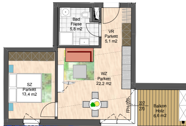
Wohnnutzfläche 46,1 m² , Balkon 7,1 m² , gesamt 53,2 m²
